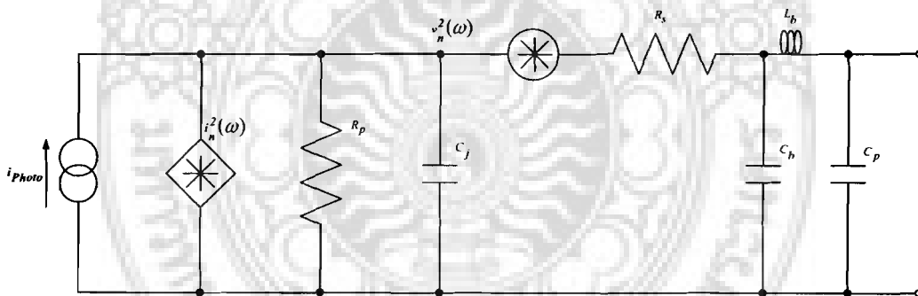
รูปที่ 2.4 สัญญาณรบกวนเชิงความร้อนที่อยู่ในโฟโตดีเทคเตอร์
