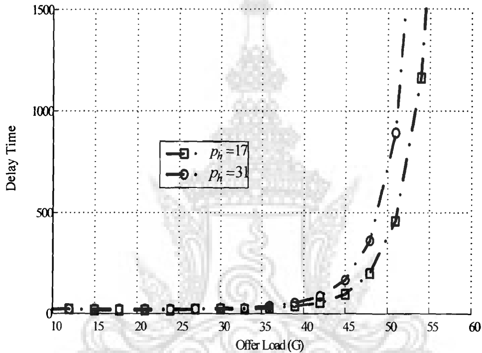
รูปที่ 5.4 ผลของหน่วงเวลาต่อค่า offer load ที่จำนวนความยาวคลื่นแสงที่วาง p_h = 17, 31 เมื่อไม่พิจารณาถึงสัญญาณรบกวนบิทน้อยส์
