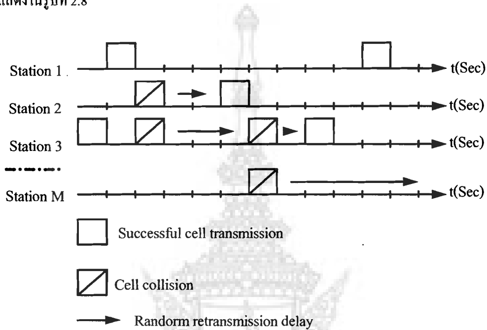
รูปที่ 2.8 กลไกการชนกันของแพ็กเก็ตเกิดในวิธีสล็อตอะโลฮ่า
