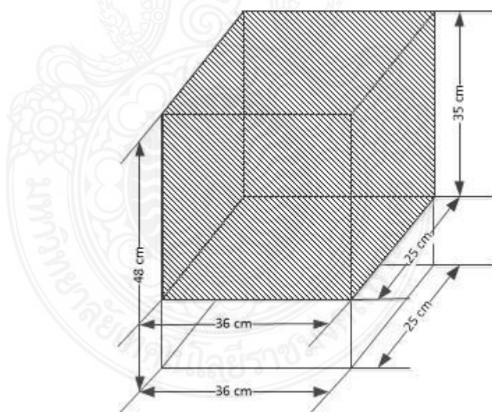
ภาพที่ 3.4 แบบแสดงขนาดก่อนและหลังการปรับปรุงแบบซ้อนทับกัน
