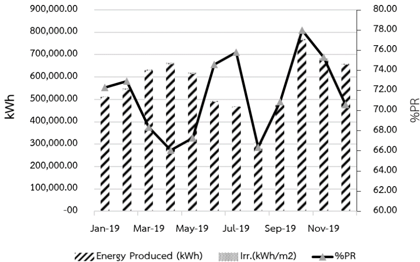
รูปที่ 9 ผลการผลิตพลังงานไฟฟ้าขนาด 5.95MWp. ปี 2562
